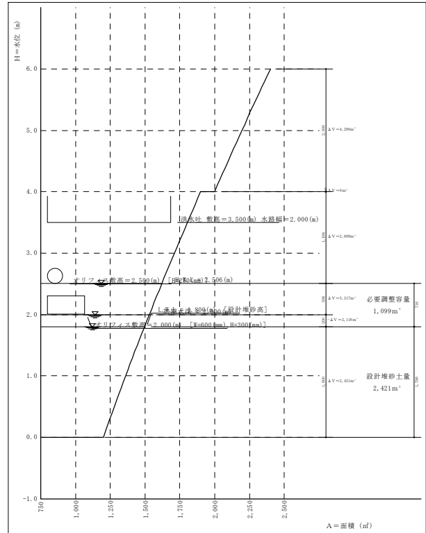
H-A 曲線
